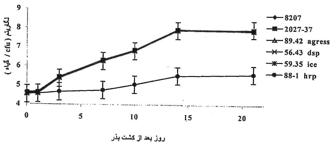
نگاره ۳. دینامیک جمعیت (جدایه ۸۲۰۷) P. s. pv. tomato (جدایه ۲۰۲۷-۳۷) P. s. pv. syringae و موتان‌های این جدایه، موتان hrp (جدایه ۸۸-۱)، موتان ice (جدایه ۵۹-۳۵)، موتاه agress (جدایه ۸۹-۴۲) و موتان dsp (جدایه ۵۶-۴۳) در گوجه فرنگی
