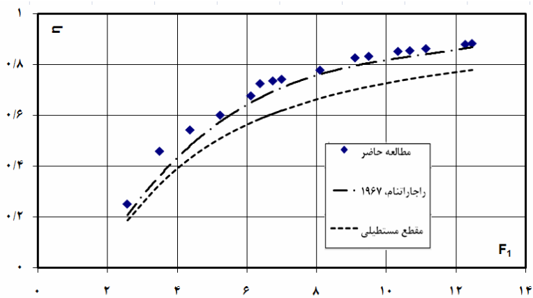
شکل ۴. تغییرات افت انرژی نسبی برحسب عدد فرود
