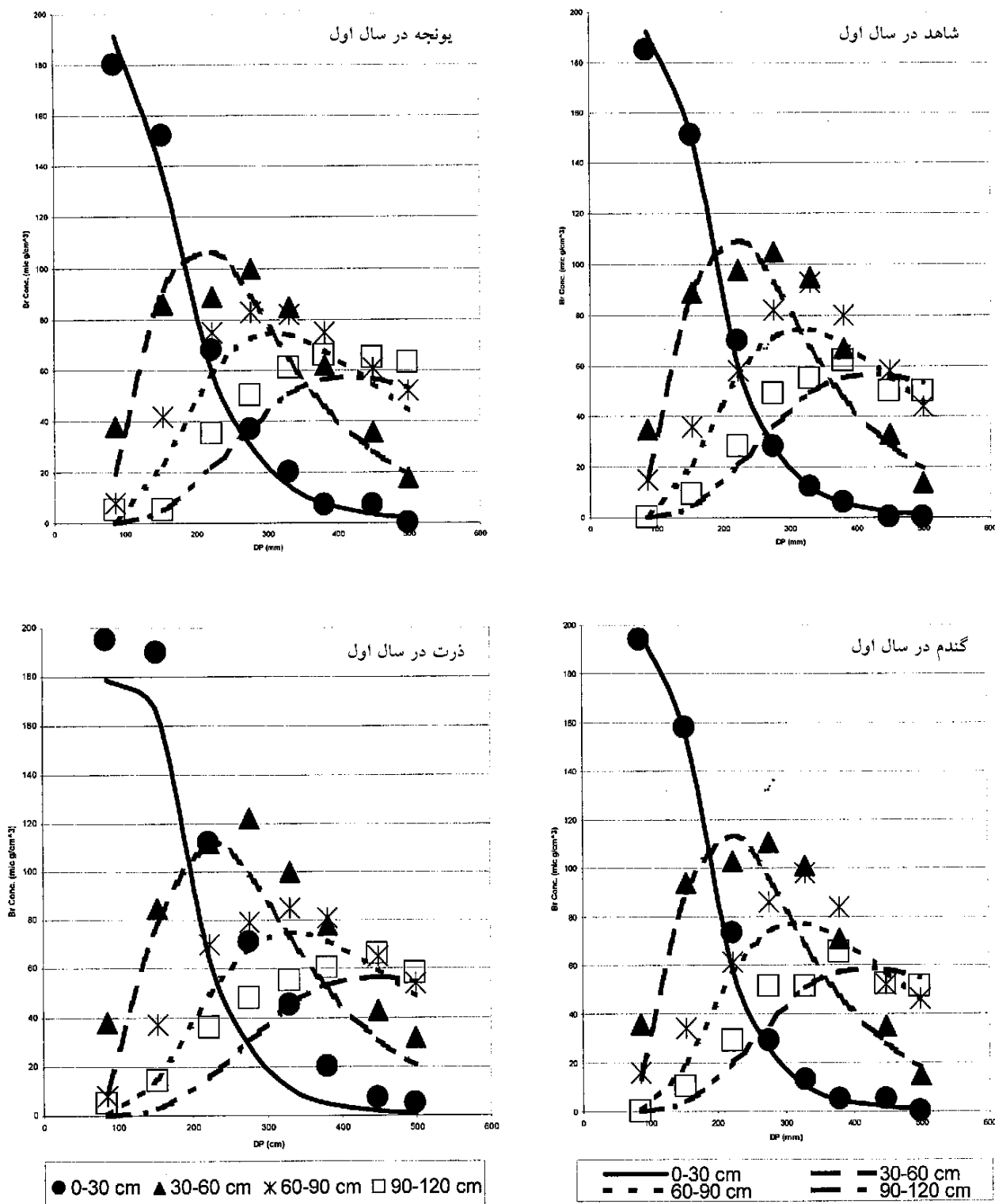
شکل ۱. غلظت‌های اندازه‌گیری شده (نشانه‌ها) و مقادیر برازش شده (خطوط) به وسیله مدل RSM در سال اول. محور افقی نمودارها مقدار نفوذ عمقی (DP) بر حسب میلی‌متر و محور عمودی غلظت برماید بر حسب میکروگرم بر سانتی‌متر مکعب خاک است.
