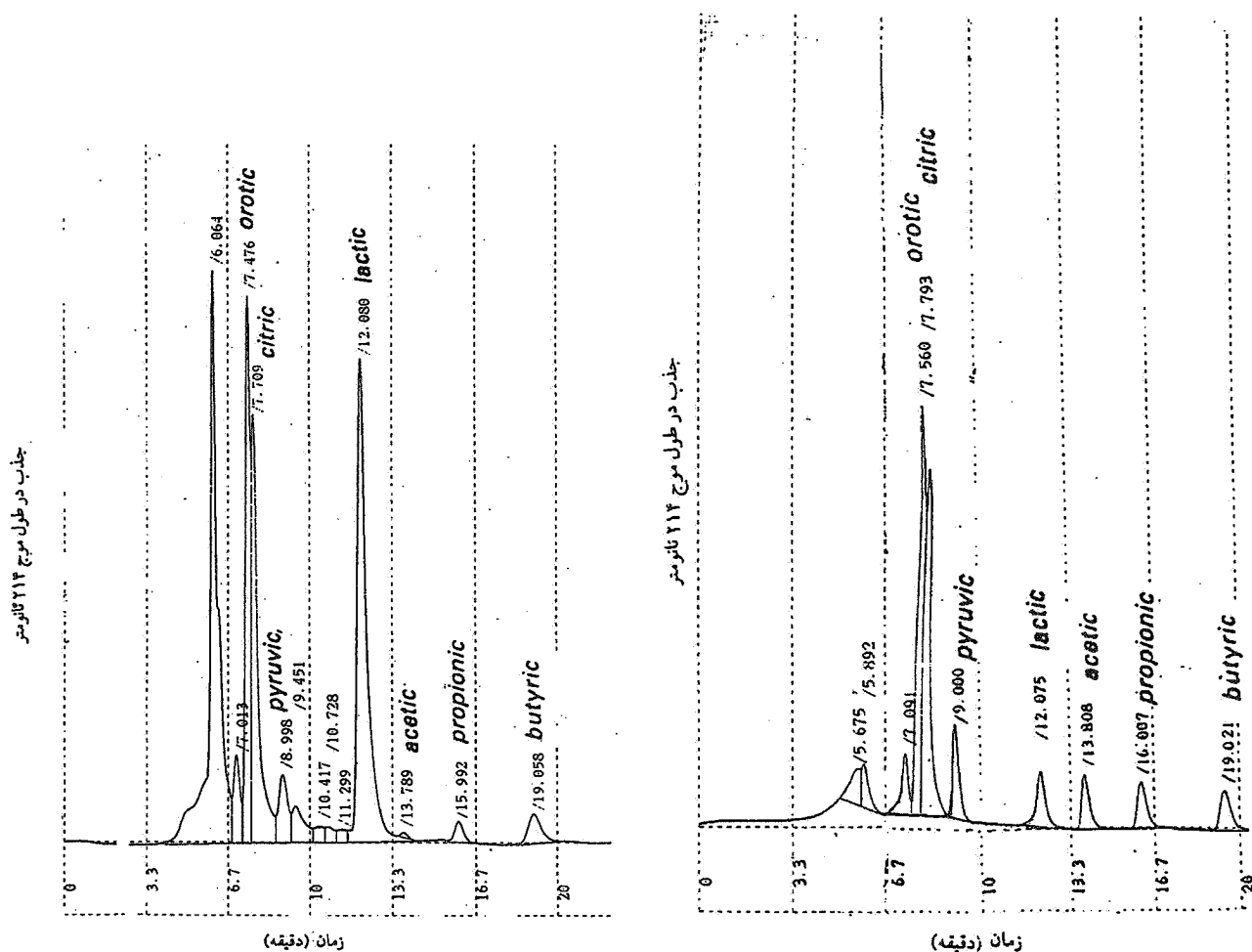
شکل ۳. کروماتوگرام HPLC اسیدهای آلی یک نمونه پنیر
