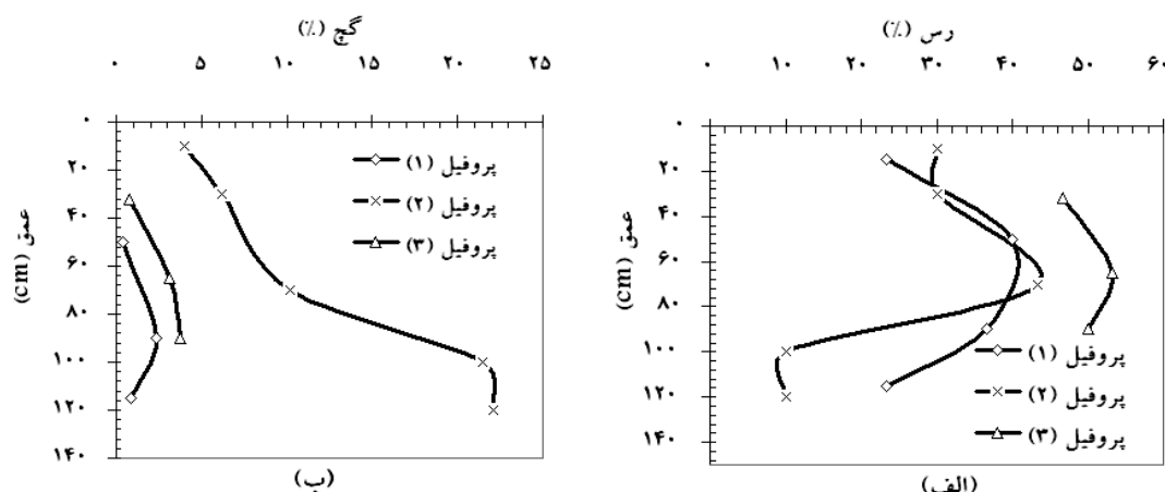
شکل ۲. الف: توزیع مقدار ذرات رس در عمق، تجمع ذرات رس در محدوده ۸۰-۶۰ عمق خاک است.
