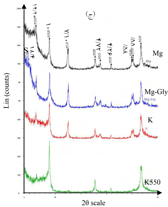
شکل ۳. نمونه‌هایی از تفرق اشعه ایکس الف: افق Byz پروفیل ۱، ب: افق Byz2 پروفیل ۲، ج: افق Byz3 پروفیل ۳، که در تیمار منیزیم گلیسرول ظهور پیک ۱۸/۴ نشانه‌ای بر وجود اسمکتیت است.
