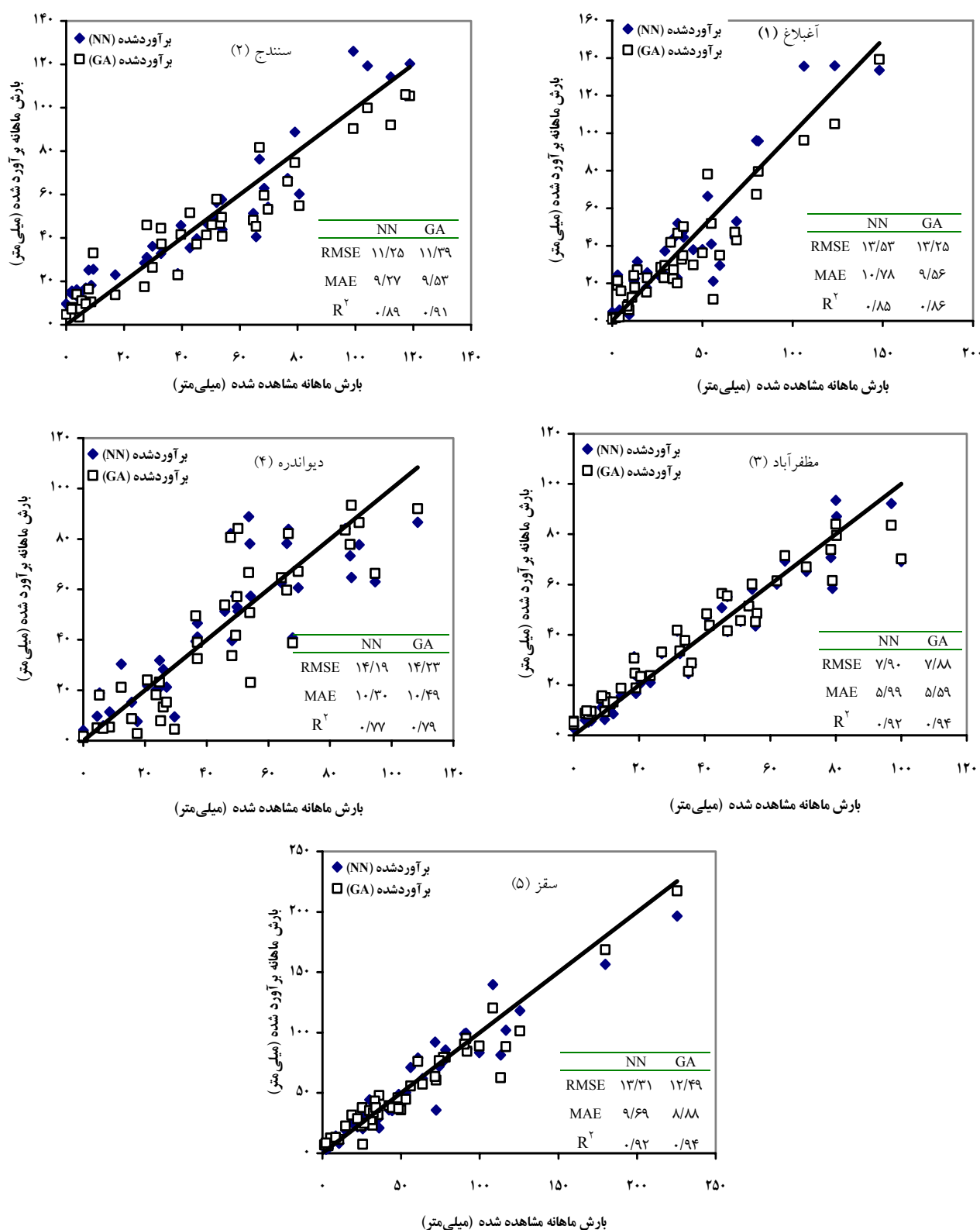
شکل ۴. پراکنش و نتایج آماری بارش ماهانه مشاهده شده و برآوردشده با استفاده از شبکه عصبی (NN) و شبکه عصبی بهینه‌سازی شده با الگوریتم ژنتیک (GA)
