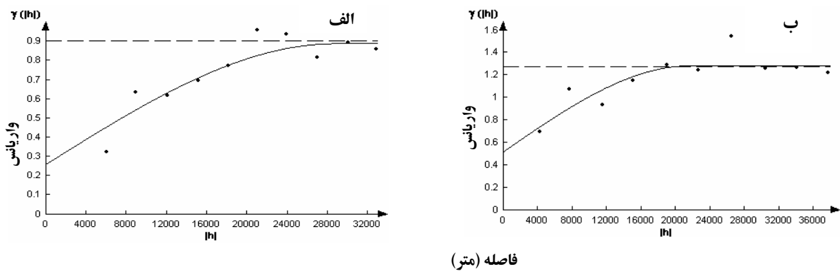
شکل ۶. واریانس جهت آرسنیک کل - الف: زاویه ۹۰ درجه (E-W) - ب: زاویه ۱۸۰ درجه (S-N)
