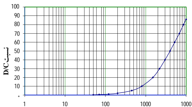
دوره برگشت اقتصادی ترین سیلاب طراحی سرریز (سال)
