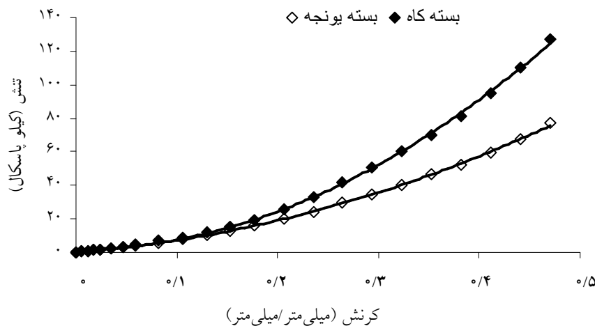
شکل ۱. نمودار مقایسه تشنش در بسته‌های یونجه و کاه در سطح گرنش طولی ۴۵٪ طول اولیه بسته‌ها
