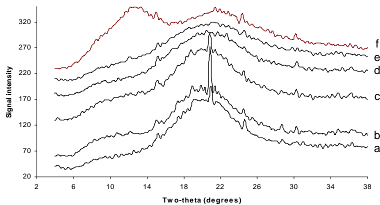
نمودار ۳. الگوی دیفرکسیون X-ray نمونه‌های انجیر تیمار یافته با ۰/۴٪ گلیسرول به تعادل رسیده در فعالیت آبی‌های مختلف (f: ۰/۸۴۳، e: ۰/۷۴۳، d: ۰/۶۴۳، c: ۰/۳۸۲، b: ۰/۲۲۷، a: ۰/۱۱۲) در دمای ۲۵ °C
