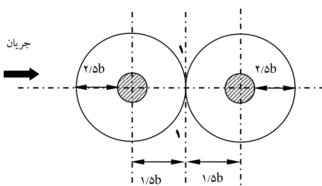
شکل ۱۶. گروه پایه دوتایی به همراه محدوده پوشش سنگ چین به صورت مقطع
