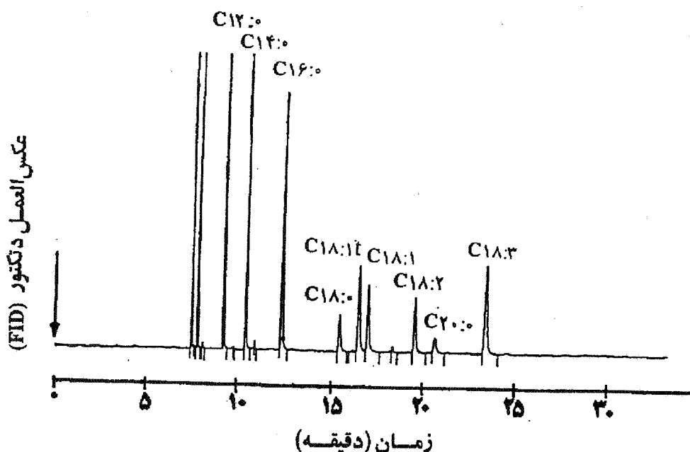
شکل ۱. نمودار کروماتوگرام گازی (GC) متیل استر اسیدهای چرب استاندارد اسیدهای چرب: لائوریک (C12:0)، میریستیک (C14:0)، پالمیتیک (C16:0)، استئاریک (C18:0)، لئوئیک (C18:1)، لینولیک (C18:2)، آراشیدیک (C20:0) و لینولیک (C18:3). با زمان ماندگاری به ترتیب ۹/۲۴، ۱۰/۳۹، ۱۲/۲۹، ۱۵/۴۱، ۱۶/۴۵، ۱۶/۹۴، ۱۹/۵۵، ۲۰/۶۴ و ۲۳/۳۸ دقیقه
