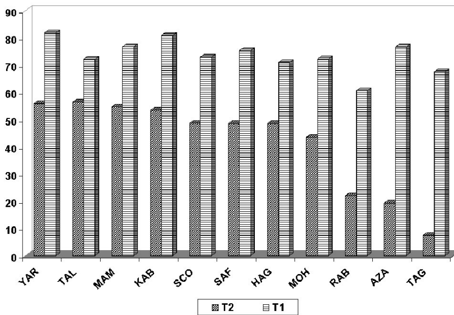
شکل ۳. مقایسه افزایش نسبی متابولیت‌های نشتی (E1) در نمونه‌های در معرض یخزدگی مصنوعی ( T_2 ) و در معرض یخزدگی طبیعی ( T_1 ) نسبت به نمونه‌های شاهد در ارقام زراعی بادام و یک گونه بادام وحشی. علائم اختصاری در جدول ۱ شرح داده شده است.
