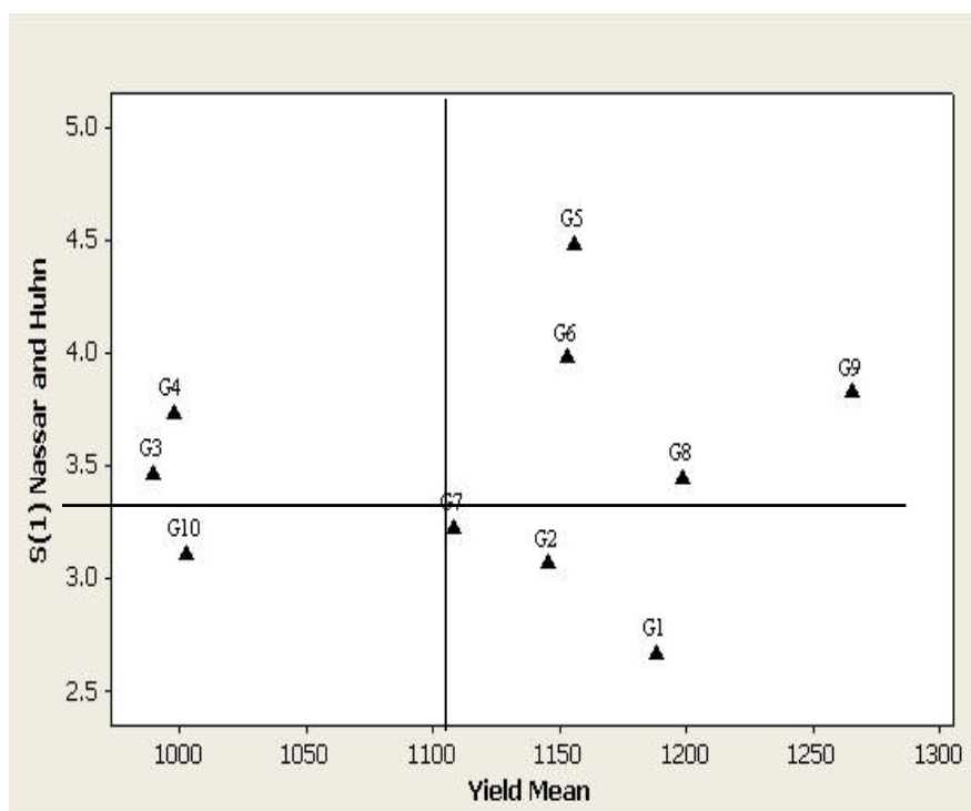
شکل ۱. نمودار پراکنش میانگین عملکرد و S_i^{(1)}
