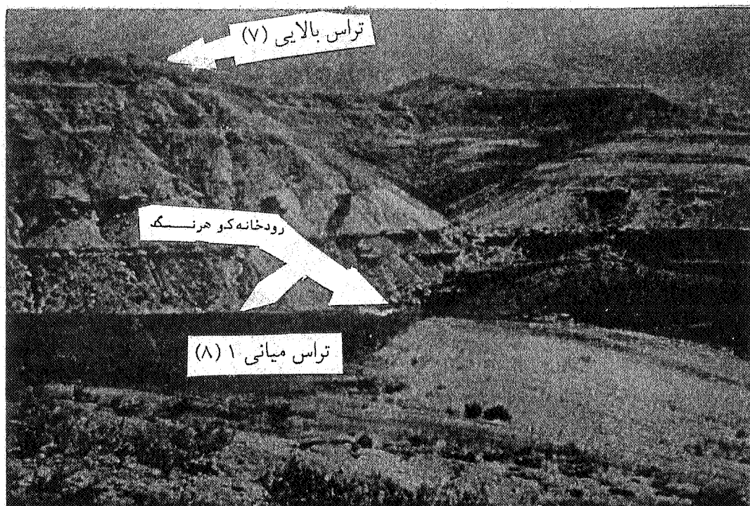
شکل ۳. نمایشی از وضع زمین‌نمای تراس‌ها در اطراف رود کوه رنگ (ناحیه اقلیمی چلگرد)
