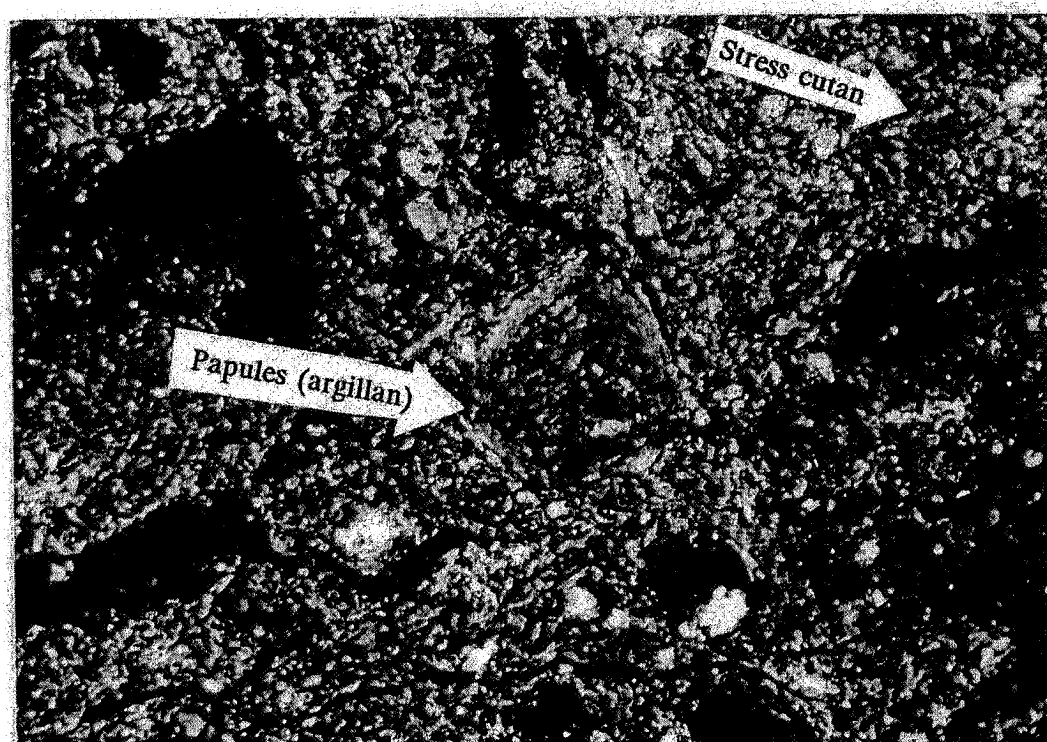
شکل ۱۰. مقطع میکروسکوپی افق 2Btkb پروفیل ۹، نور پلاریزه، طول عکس برابر ۰/۵ میلی متر [آرجیلان با منشأ رسوبی (بایبول) و کوتان فشاری به صورت غالب را نشان می دهد.]
