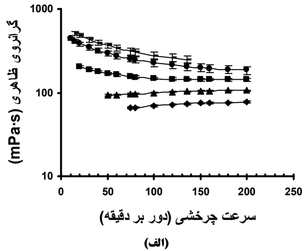
شکل ۲. نمایش رفتار جریان محلول‌های پودر ثعلب در غلظت‌های مختلف (۶، ۵، ۴، ۳، ۲ گرم در لیتر) در دمای ۲۵ درجه سانتی‌گراد و پ هاش ۷ (الف) سرعت چرخشی در مقابل گرانیوی ظاهری (ب) سرعت برشی در مقابل گرانیوی ظاهری.
