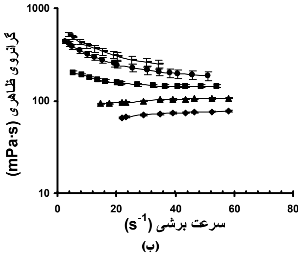
شکل ۲. نمایش رفتار جریان محلول‌های پودر ثعلب در غلظت‌های مختلف (۶، ۵، ۴، ۳، ۲ گرم در لیتر) در دمای ۲۵ درجه سانتی‌گراد و پ هاش ۷ (الف) سرعت چرخشی در مقابل گرانیوی ظاهری (ب) سرعت برشی در مقابل گرانیوی ظاهری.
