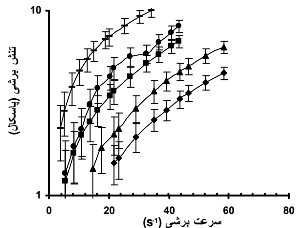
شکل ۳. نمایش تغییرات سرعت برشی در مقابل تنش برشی در محلول‌های پودر ثعلب در غلظت‌های مختلف (۶، ۵، ۴، ۳، ۲ گرم در لیتر) در دمای ۲۵ درجه سانتی‌گراد و پ هاش ۷.
