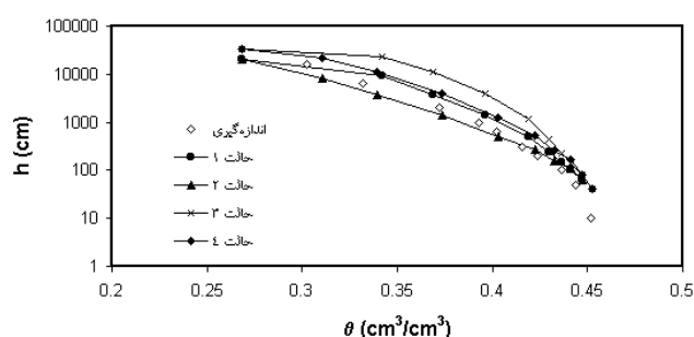
شکل ۱. منحنی مشخصه آب خاک برای چهار حالت مختلف و مقایسه با منحنی اندازه‌گیری شده در خاک شماره ۱ (بافت رس)
