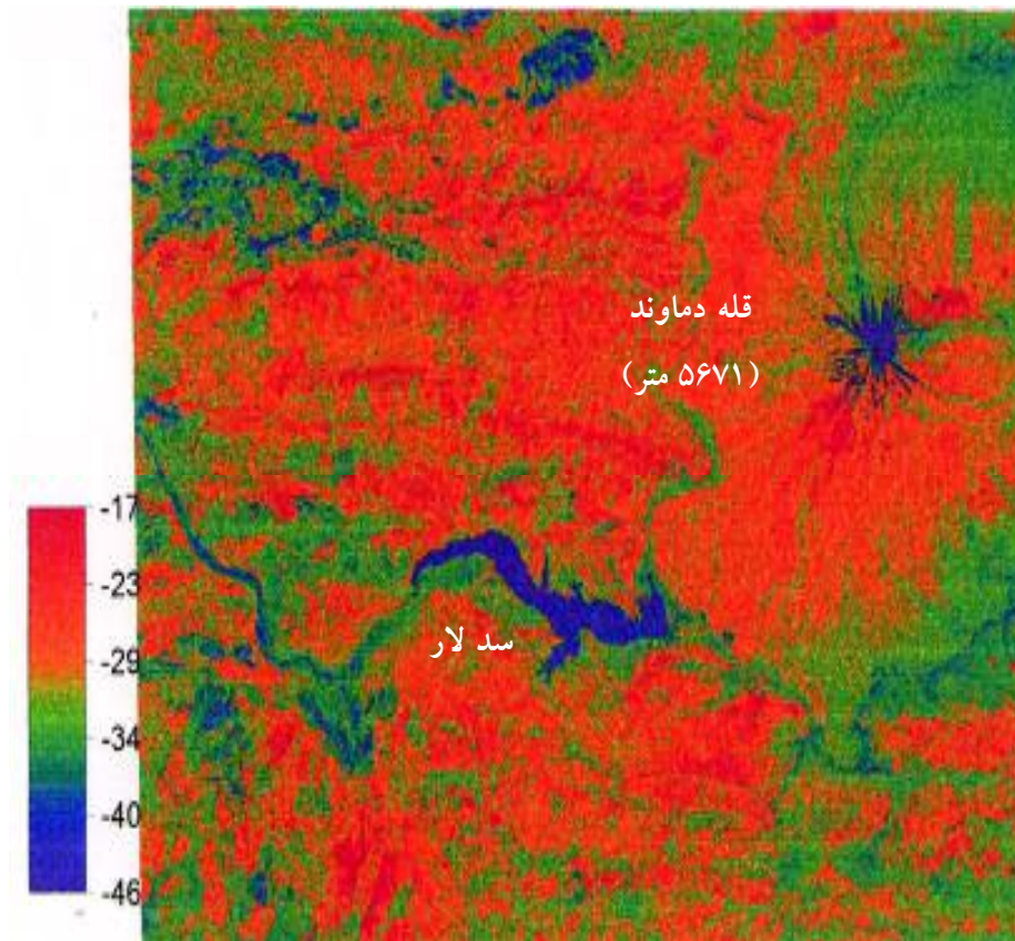
شکل ۳. تصویر ماهواره‌ای تصحیح شده (محدوده ۱۷ تا ۲۹ = بدون پوشش گیاهی، ۳۴ = پوشش مرتعی، ۴۰ - برف و ۴۶ - آب).
