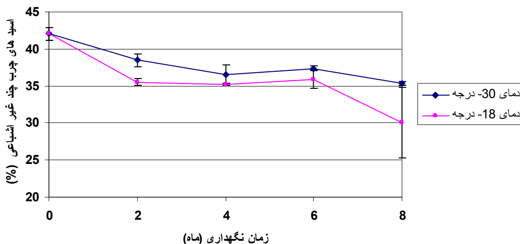
شکل ۲. تغییرات اسیدهای چرب چند غیر اشیباعی ماهی کیلکای آنچوی در زمان‌ها و دماهای مختلف نگهداری
