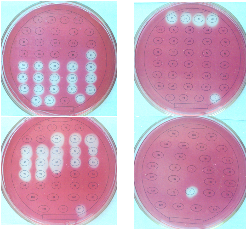
شکل ۳. بررسی فعالیت آنزیم پلی گالاتوروناز به روش test plate :
