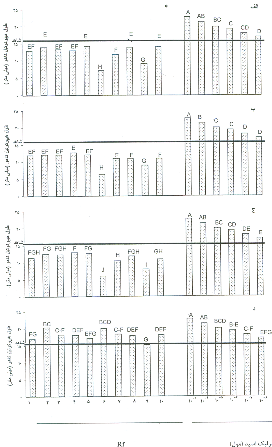
شکل ۳. واکنش هیپوکوتیل های کاهو به غلظت های مختلف اسید جیبرلیک و عصاره حاصل از قسمت های مختلف بذر رقم آرکینین
