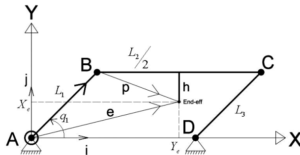
شکل ۸. بردار مکان پنجه
