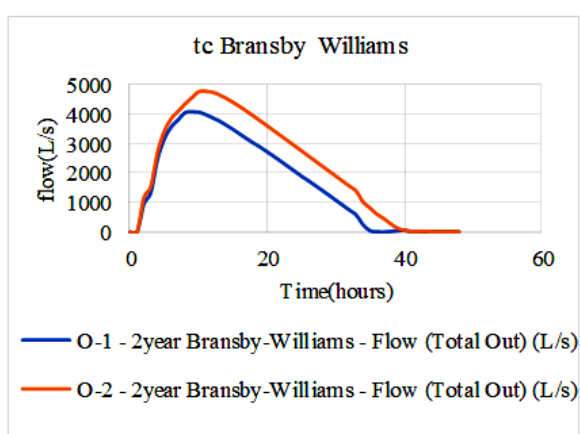
شکل ۶. هیدروگراف خروجی سیلاب شبیه‌سازی سناریوی ۲ زیرحوضه با دوره بازگشت ۲ ساله و با روش‌های مختلف محاسبه زمان تمرکز
