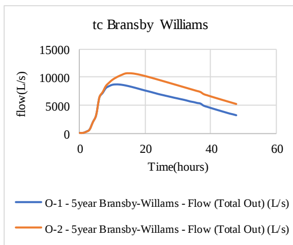
شکل ۸. هیدروگراف خروجی سیلاب شبیه‌سازی سناریوی ۲ زیرحوضه با دوره بازگشت ۵ ساله و با روش‌های مختلف محاسبه زمان تمرکز
