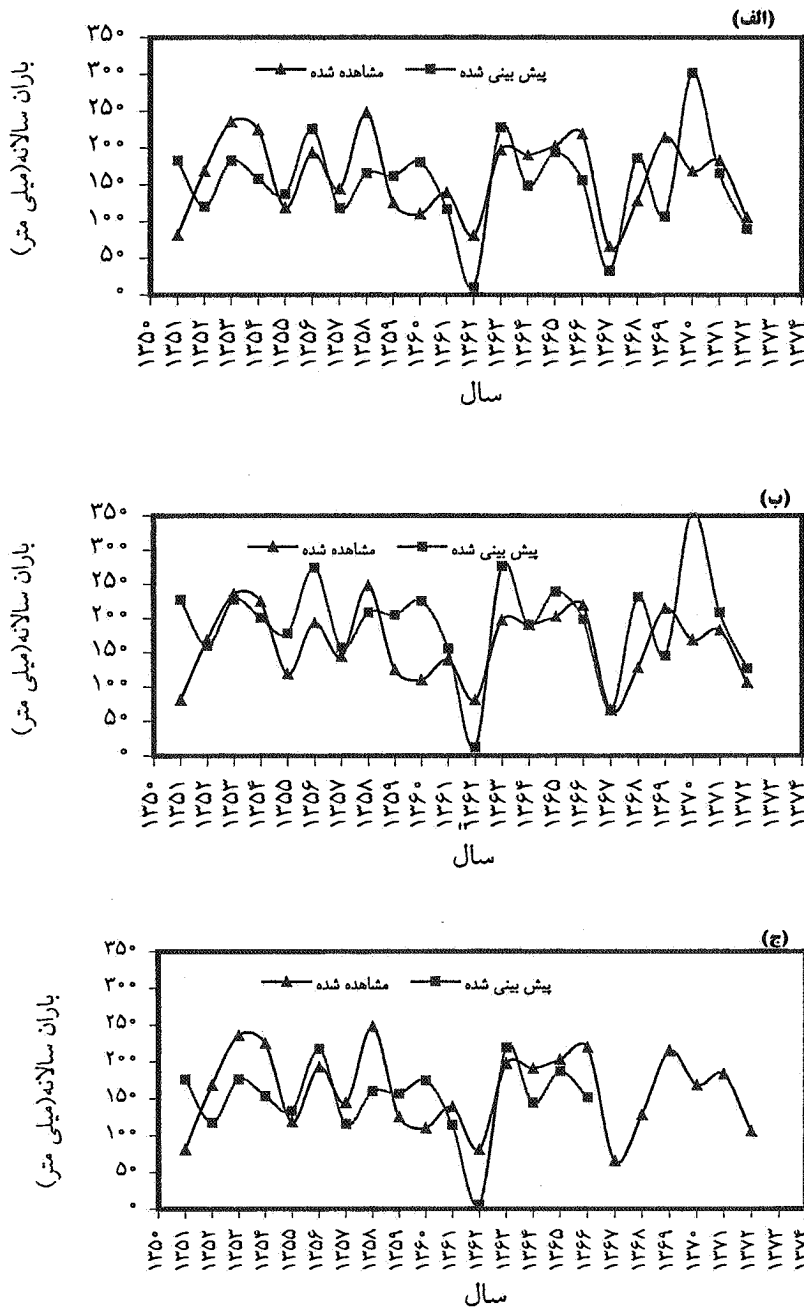
شکل ۵. مقادیر مشاهده‌ای و پیش بینی شده بارندگی سالانه الف- مدل (۲) ب- مدل (۷) ج- مدل (۸)
