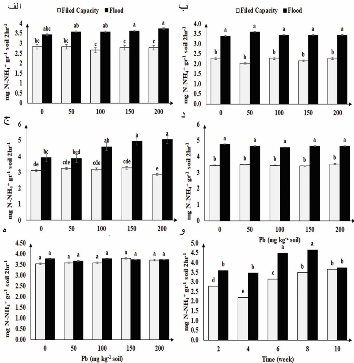
شکل ۱. تغییرات فعالیت آنزیم اوره‌آز در طی: الف) دو، ب) چهار، ج) شش، د) هشت، ه) ده هفته انکوباسیون خاک در دو رژیم متفاوت آبی و (و) تغییرات آن در طی زمان است. (مقادیر، میانگین سه تکرار \pm SD است. حروف مشابه در هر نمودار بیانگر عدم تفاوت معنی‌دار بین تیمارها با آزمون توکی در سطح ۵ درصد است).
