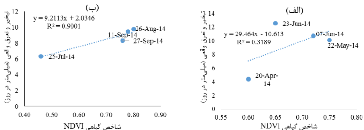
شکل ۱۳. ارتباط مقادیر NDVI-ET c در زمین شماره سه در سال ۲۰۱۴: الف) کشت اول و ب) کشت دوم
