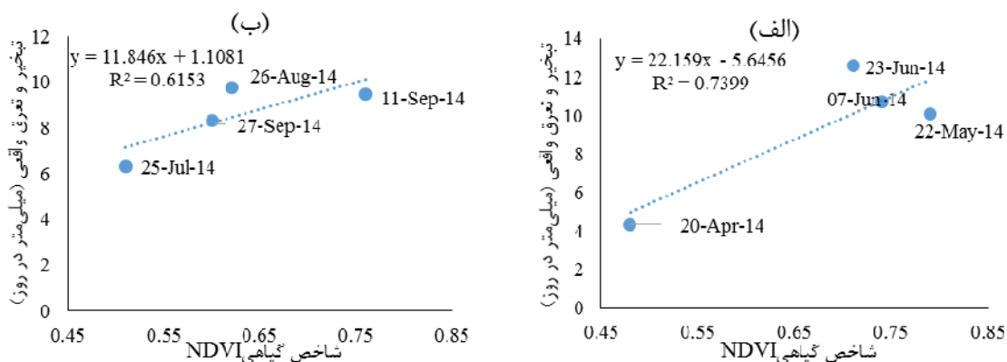
شکل ۱۷. ارتباط مقادیر NDVI-ET c در زمین شماره پنج در سال ۲۰۱۳: الف) کشت اول و ب) کشت دوم
