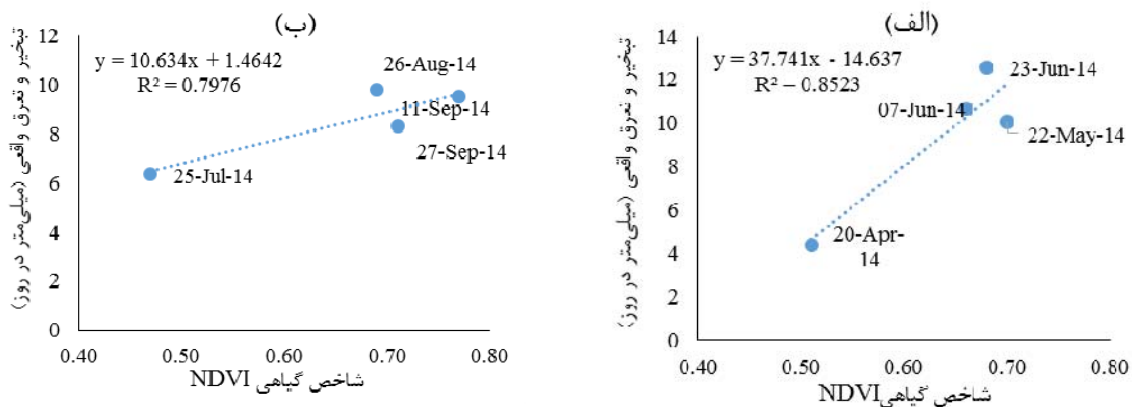
شکل ۱۱. ارتباط مقادیر NDVI-ET c در زمین شماره دو در سال ۲۰۱۴: الف) کشت اول و ب) کشت دوم
