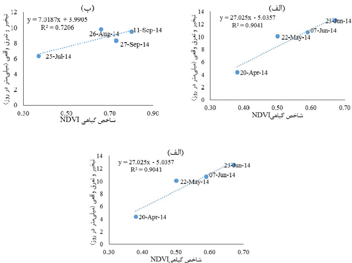
شکل ۱۸. ارتباط مقادیر NDVI-ET c در زمین شماره شش در سال ۲۰۱۴: الف) کشت اول و ب) کشت دوم
