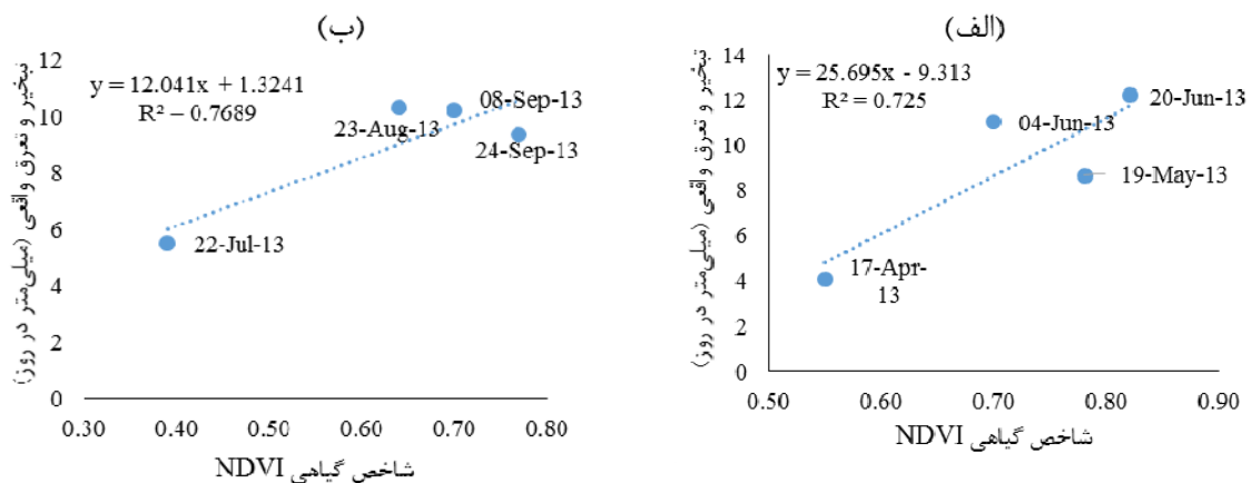
شکل ۱۲. ارتباط مقادیر NDVI-ET c در زمین شماره سه در سال ۲۰۱۳: الف) کشت اول و ب) کشت دوم
