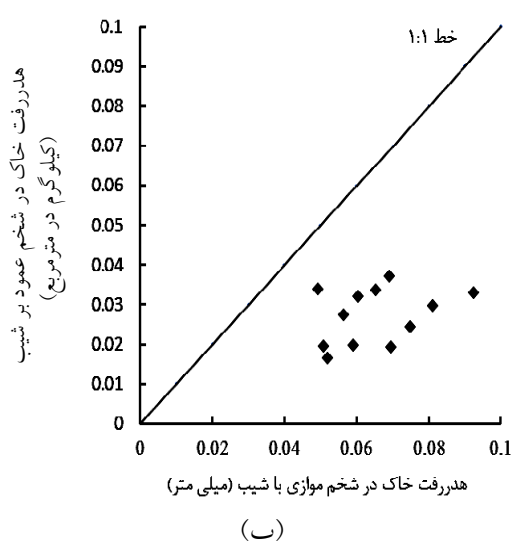
شکل ۳. مقایسه بین دو جهت خاک‌ورزی (روی خط تراز و موازی شیب) از نظر هدررفت آب (الف) و هدررفت خاک (ب)
