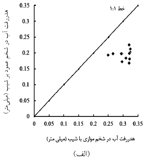
شکل ۳. مقایسه بین دو جهت خاک‌ورزی (روی خط تراز و موازی شیب) از نظر هدررفت آب (الف) و هدررفت خاک (ب)
