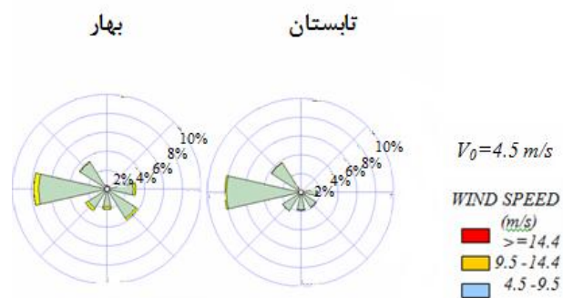
شکل ۲. گل طوفان‌های فصلی (تابستان و بهار) ایستگاه سینوپتیک کرمانشاه (۱۹۸۶-۲۰۰۶)
