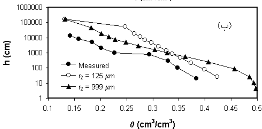
شکل ۶. منحنی مشخصه آب خاک بر مبنای \alpha محاسبه شده از روش لاجستیک (الف) و خطی (ب) و مقایسه با منحنی مشاهده‌ای در خاک ملاثانی (لوم)
