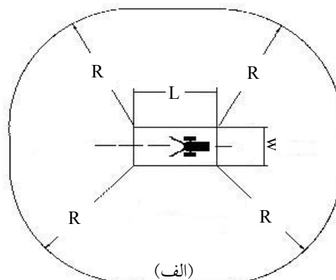
شکل ۱ (الف) ابعاد ناحیه اندازه‌گیری صدا (ب) تراکتور دوچرخ و تجهیزات اندازه‌گیری صدا در موقعیت گوش راننده
