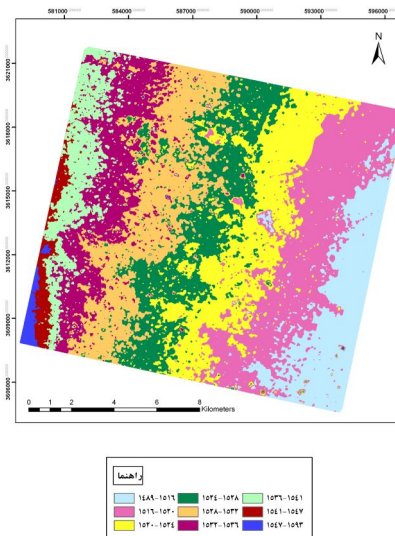
شکل ۳. طبقه بندی مدل رقومی ارتفاعی در ۹ لایه ارتفاعی با روش NaturalBreaks بر حسب متر
