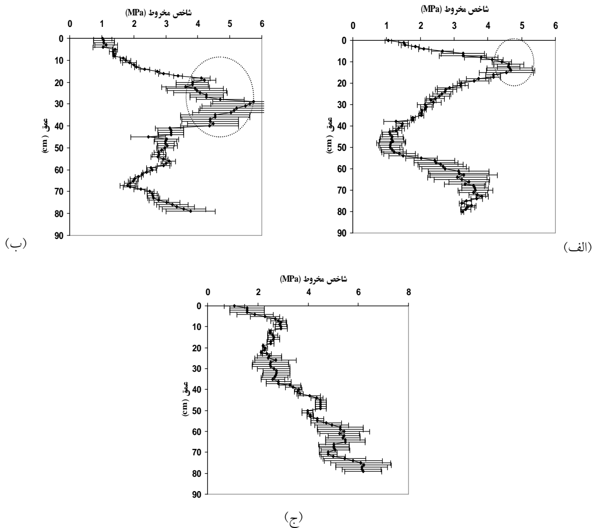
شکل ۶. تغییرات میانگین مقاومت مکانیکی (شاخص مخروط) خاک با عمق برای بافت‌های: (الف) لوم شنی با درصد رطوبت وزنی و چگالی ظاهری خاک رویین به ترتیب برابر ۱۲/۴ و ۱/۶۸ مگاگرم بر متر مکعب، (ب) لوم رسی با درصد رطوبت وزنی و چگالی ظاهری خاک رویین به ترتیب برابر ۱۵/۹ و ۱/۶۸ مگاگرم بر متر مکعب و (ج) رسی با درصد رطوبت وزنی و چگالی ظاهری خاک رویین به ترتیب برابر ۱۵/۴ و ۱/۵۰ مگاگرم بر متر مکعب. مقادیر رطوبت وزنی خاک زیرین به ترتیب برابر ۱۳/۶، ۱۷/۶ و ۱۵/۵ درصد بود. این مزارع تحت بازرویی دوم بودند. میله‌های افقی بیانگر \pm یک خطای معیار می‌باشند. دایره‌های خط چین محدوده سخت لایه‌ها را نشان می‌دهند
