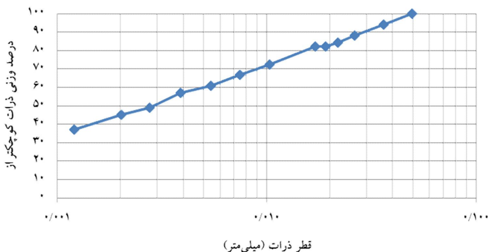
شکل ۱. منحنی دانه‌بندی خاک رس کهریزک
