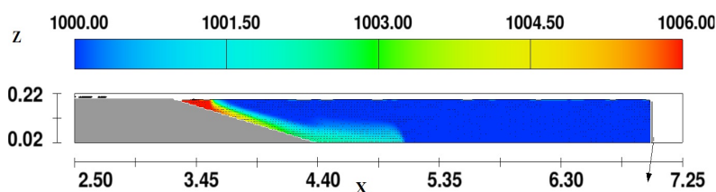
شکل ۹. نتایج مدل ریاضی تحت شرایط مدل تلاطمی RNG برای آزمایش ( \rho = 1006 \frac{\text{kg}}{\text{m}^3} , S = 16\% , Q = 1/9 \text{ L/s} )
