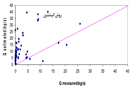
شکل ۳. مقایسه بین باربستر محاسبه شده و اندازه گیری شده
