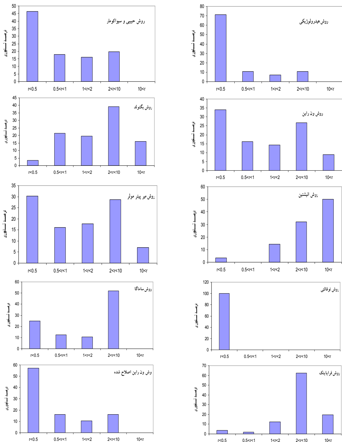
شکل ۴. تغییرات بازه‌های نسبت نایجوری بر حسب درصد فراوانی برای برآورد بار بستر براساس فرمول‌های مختلف
