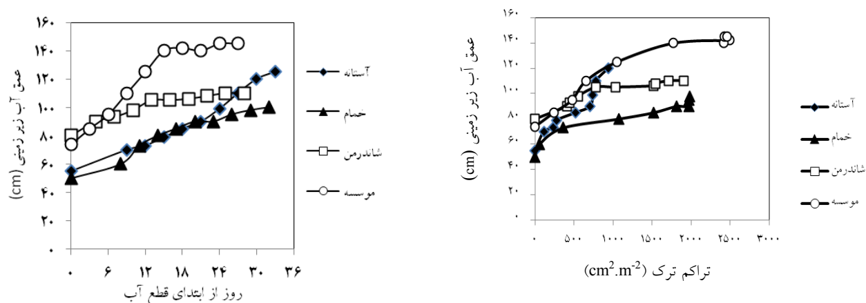
شکل ۴. تغییرات عمق ترک زیرزمینی در خاک‌های مطالعه شده نسبت به زمان و تراکم ترک
