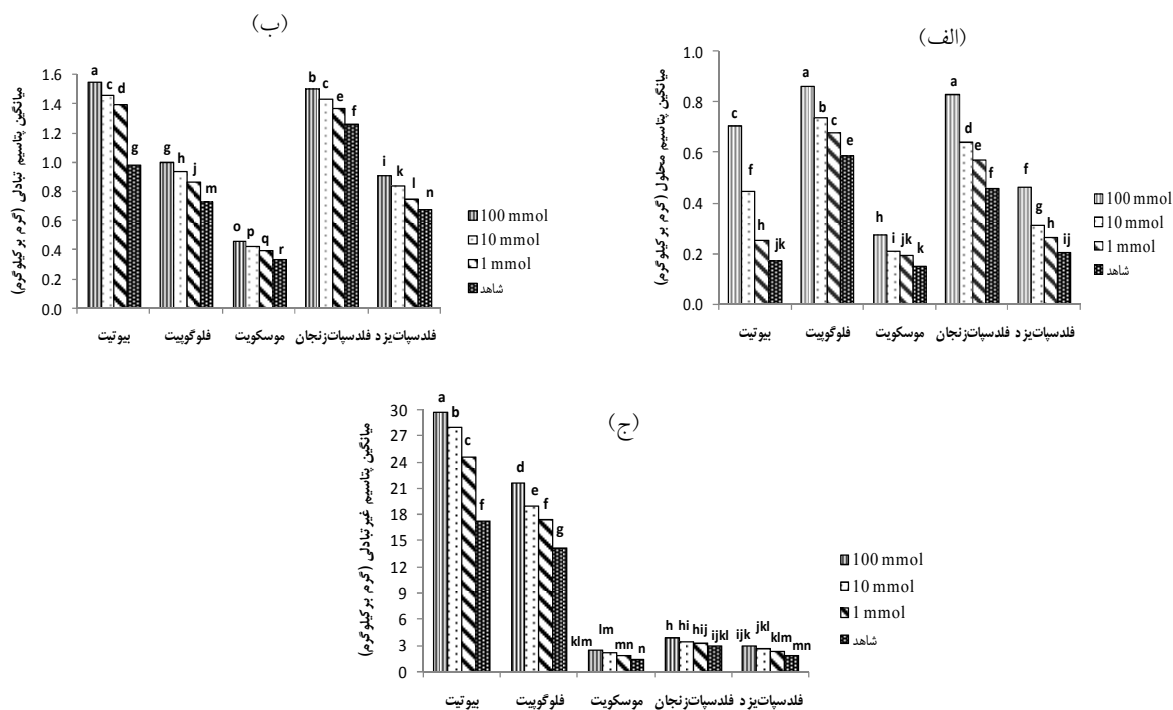
شکل ۱. میانگین پتاسیم محلول (الف)، تبادلی (ب) و غیر تبادلی (ج) آزاد شده تحت تأثیر اسید اگزالیک با غلظت‌های مختلف در کانی‌های بیوتیت، فلوگویت، موسکویت، فلدسپات زنگان و فلدسپات یزد (میانگین‌های دارای حرف مشترک در سطح ۵٪ دارای اختلاف معنی‌دار نمی‌باشند)
