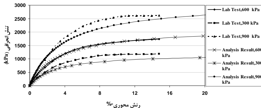
شکل ۴. نتایج کالیبراسیون مصالح هسته سد، M_2 ، با مدل الاستیک غیرخطی و مقایسه نتایج تنش انحرافی - کرنش محوری بین مدل و نتایج آزمایشگاه در مصالح هسته در شرایط CD
