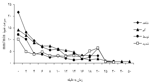
ج) سرعت نفوذ در شدت ترافیک‌های مختلف در مسیر چوبکشی ۱-۱۵ سال
