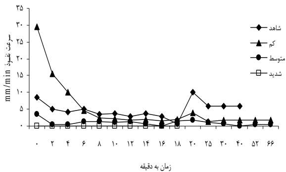
الف) سرعت نفوذ در شدت ترافیک‌های مختلف در مسیر چوبکشی ۱-۵ سال
