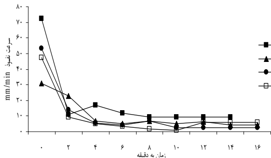
د) سرعت نفوذ در شدت ترافیک‌های مختلف در مسیر چوبکشی ۱۵-۲۰ سال
