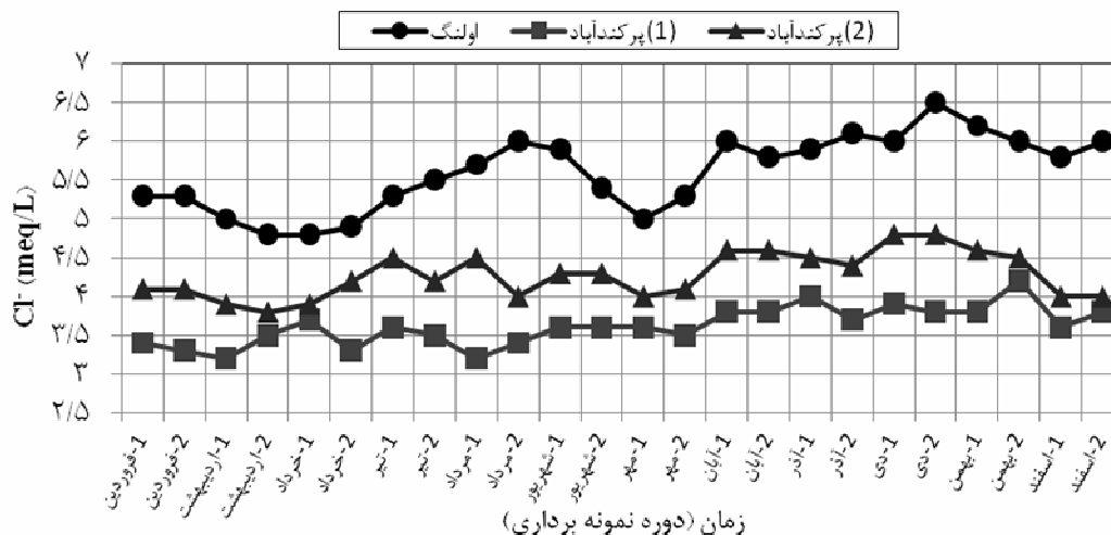
نمودار ۳. تغییرات سالیانه غلظت یون کلراید در پساب تصفیه‌خانه‌های فاضلاب شهر مشهد
