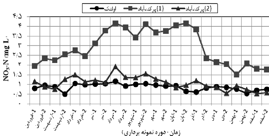
نمودار ۵. تغییرات سالیانه نیتروژن نیتروژن در پساب تصفیه‌خانه‌های فاضلاب شهر مشهد
