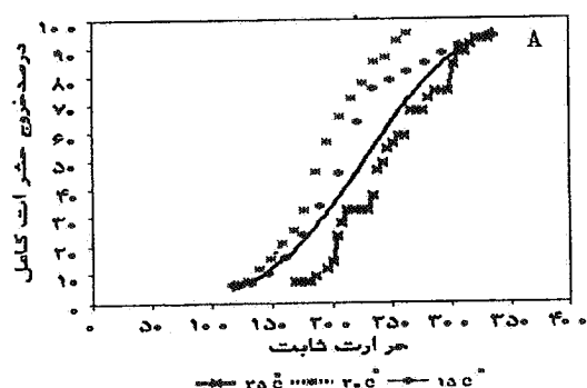
شکل ۵. درصد پیدایش حشرات کامل زنبور سیاه مغزخوار پسته و دمای یک‌نواخت لازم از زمان تشکیل ۵۰٪ شفیره تا پیدایش حشرات کامل آن. الف) شرایط آزمایشگاهی، ب) شرایط صحرایی
