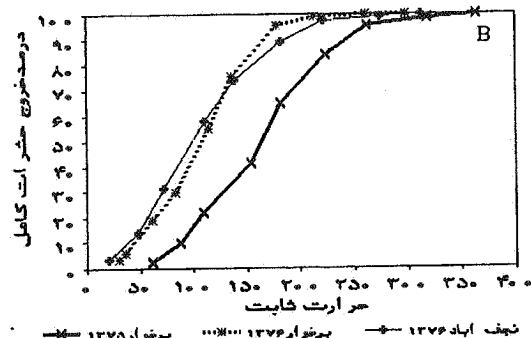
شکل ۳. دمای یک‌نواخت لازم برای درصدهای پیدایش حشرات کامل زنبور سیاه مغزخوار پسته، از زمان تشکیل ۵۰٪ شفیره آن بر پایه آستانه کمترین دمای ۱۱ درجه سانتی‌گراد. الف) شرایط آزمایشگاهی، ب) شرایط صحرایی
