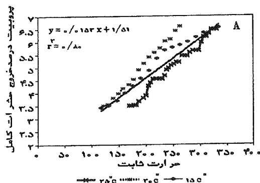
شکل ۳. دمای یک‌نواخت لازم برای درصدهای پیدایش حشرات کامل زنبور سیاه مغزخوار پسته، از زمان تشکیل ۵۰٪ شفیره آن بر پایه آستانه کمترین دمای ۱۱ درجه سانتی‌گراد. الف) شرایط آزمایشگاهی، ب) شرایط صحرایی
