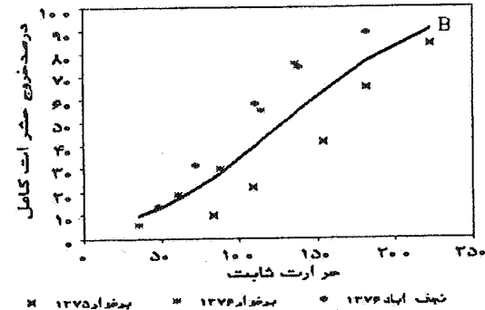
شکل ۵. درصد پیدایش حشرات کامل زنبور سیاه مغزخوار پسته و دمای یک‌نواخت لازم از زمان تشکیل ۵۰٪ شفیره تا پیدایش حشرات کامل آن. الف) شرایط آزمایشگاهی، ب) شرایط صحرایی
