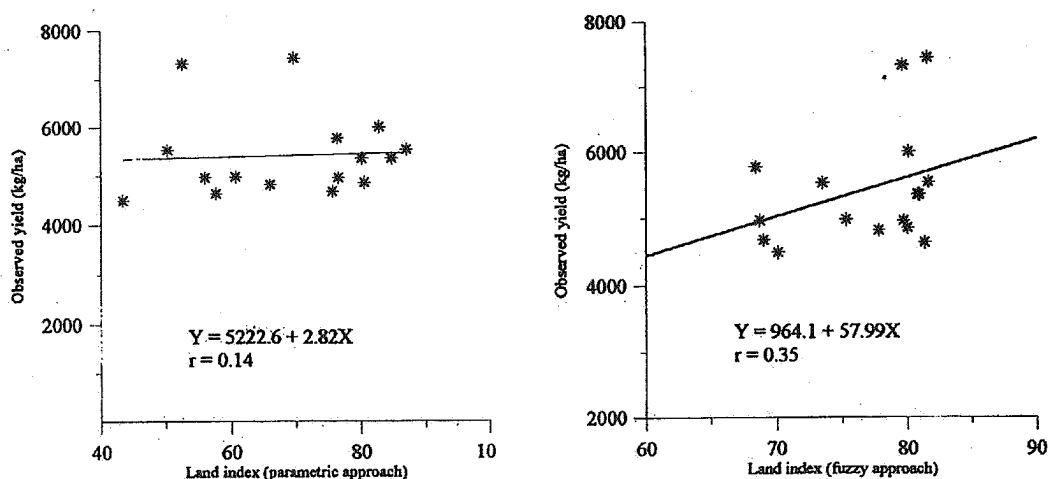
شکل ۴. خط برگشت و هم‌بستگی بین شاخص اراضی به دست آمده از روش پارامتریک (چپ) و روش فازی (راست) و عملکرد مشاهده شده گندم آبی. مدل‌ها به همراه ضرایب آنها روی نمودار نشان داده شده است.
