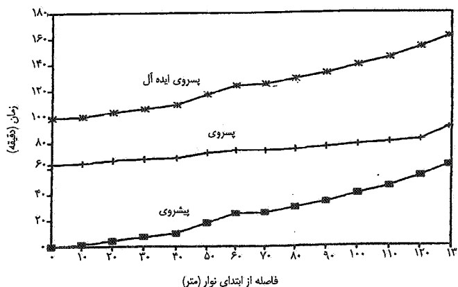
شکل ۴- منحنیهای پیشرویی، پسروی و پسروی ایده آل برای یکی از مزارع یونجه در شهرستان گچساران
