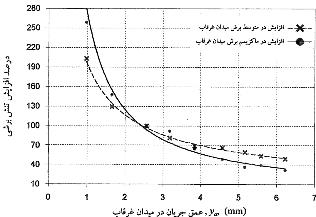
شکل ۳. افزایش در میزان متوسط و حداکثر تنش برشی میدان غرقاب به واسطه تداخل جریان‌های مجرای اصلی و میدان غرقاب، که به صورت درصد مقادیر نسبت به حالت جریان نامداخل ارائه شده است (۱۹).
