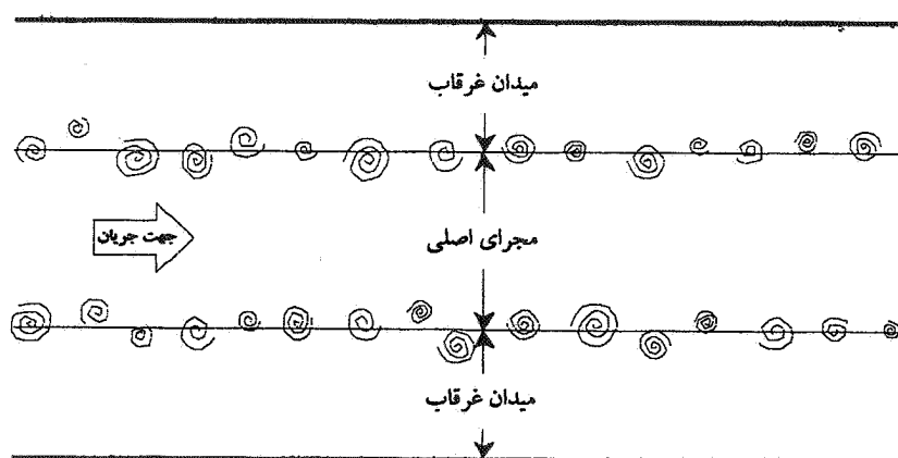
شکل ۲. ردیف گرداب‌های ایجاد شده در محل اتصال میدان غرقاب به مجرای اصلی
