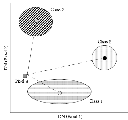
شکل ۱. تجسم شمایک طبقه بندی کننده حداقل فاصله از میانگین
