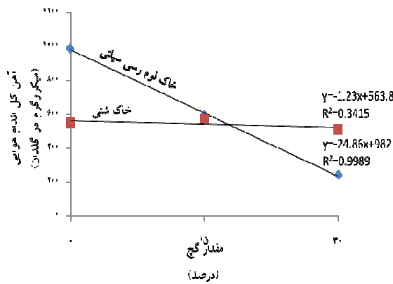
شکل ۳. اثر مقادیر مختلف گچ بر جذب آهن کل اندام هوایی توسط ذرت در دو نوع بافت خاک (هر نقطه میانگین ۹ داده است).
