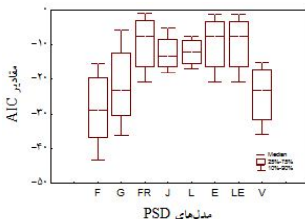
شکل ۳. نمودارهای جعبه‌ای مقادیر AIC در ۷۱ خاک مورد مطالعه. (F = مدل فردلاند، G = مدل گمپرتز، FR = مدل فراکتال، J = مدل جیکی، L = مدل لگاریتمی، E = مدل نمایی، LE = مدل لگاریتمی - نمایی و V = مدل ون‌گونختن)
