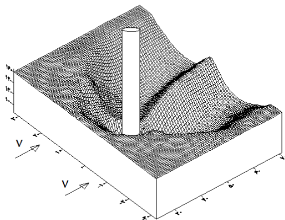
شکل ۶. توپوگرافی حفره آبستگي آزمایش G_1
