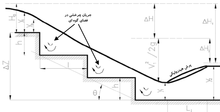
شکل ۳. معرفی شیب شکن پلکانی و اجزای هندسی و هیدرولیکی آن
